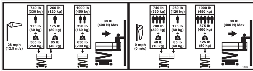
S3370RT
